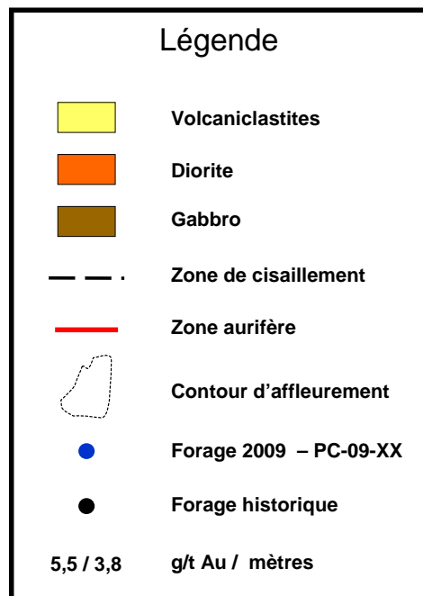
Figure 2: Géologie et forages sur l'indice Highway
